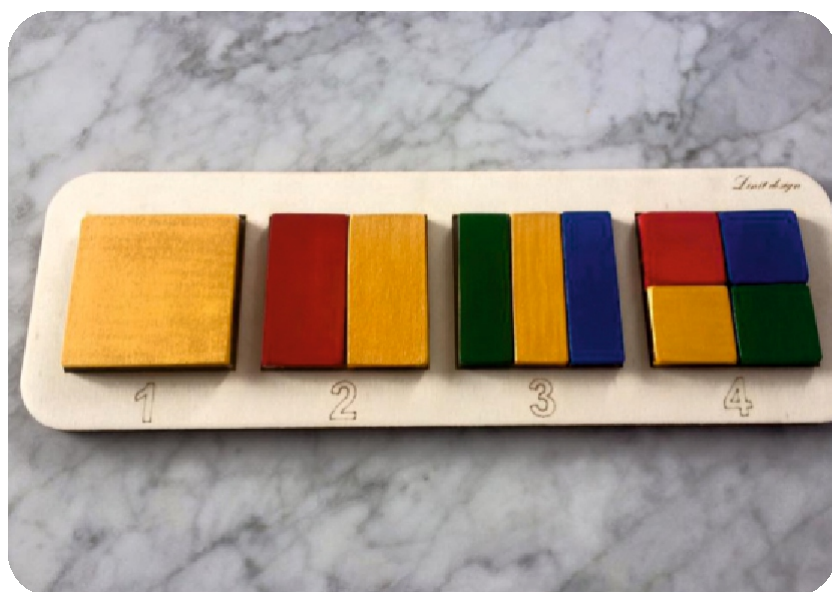
DIJELOVI KVADRATA
