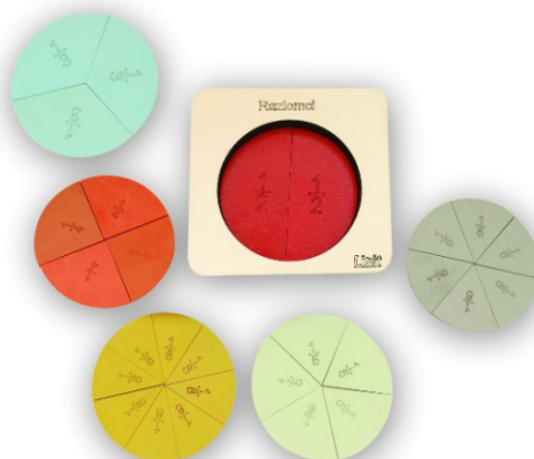
RAZLOMCI
