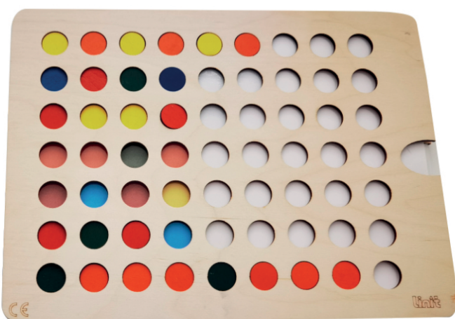
LOGIČKI SLIJED
